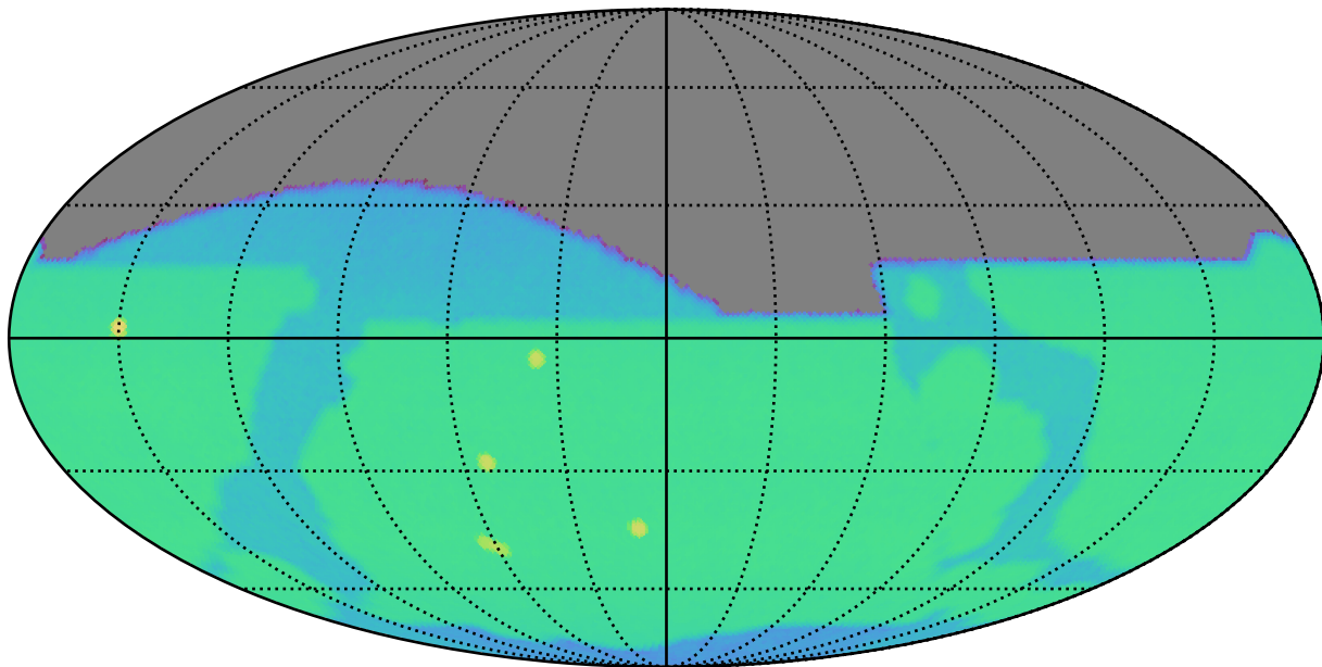
weather_cloudso18v3.4_10yrs i: SurfaceBrightLimit
