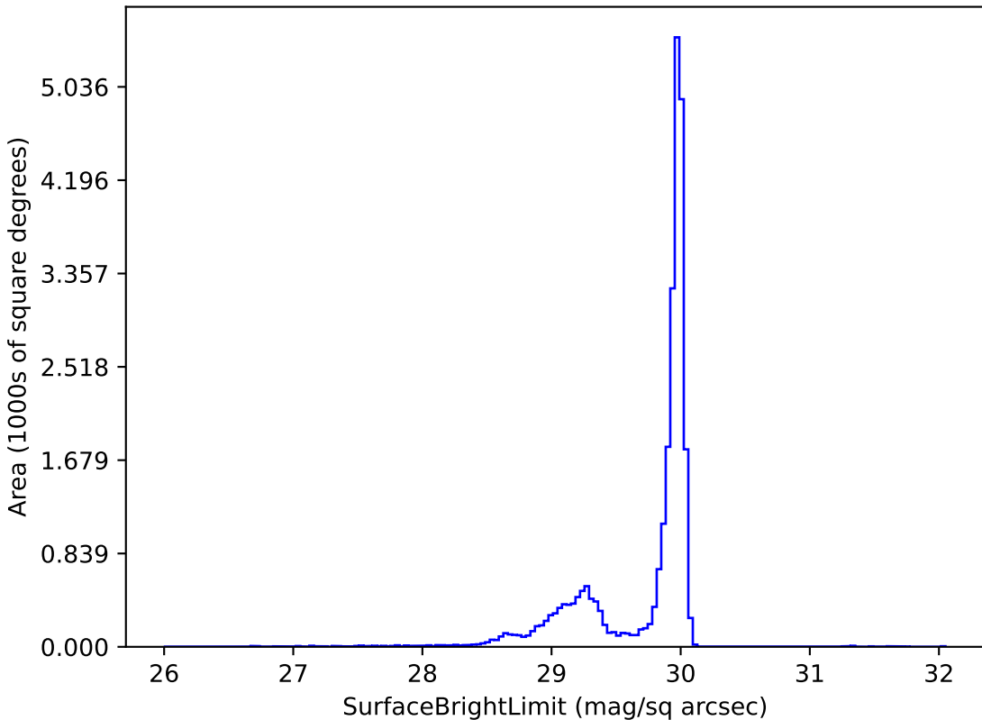
weather_cloudso18v3.4_10yrs i: SurfaceBrightLimit
