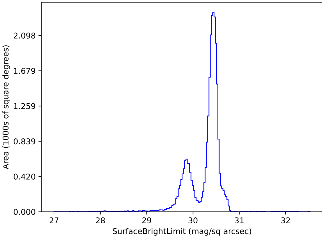
weather_cloudso18v3.4_10yrs g: SurfaceBrightLimit
