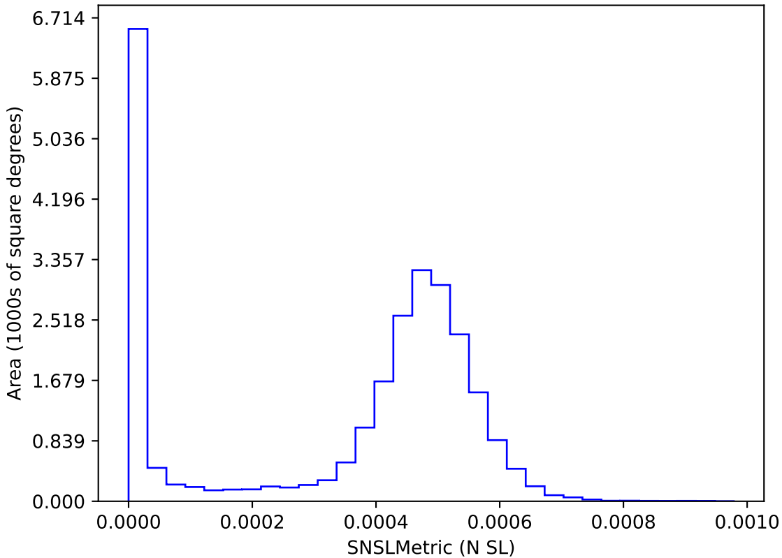
weather_cloudso18v3.4_10yrs : SNSLMetric
