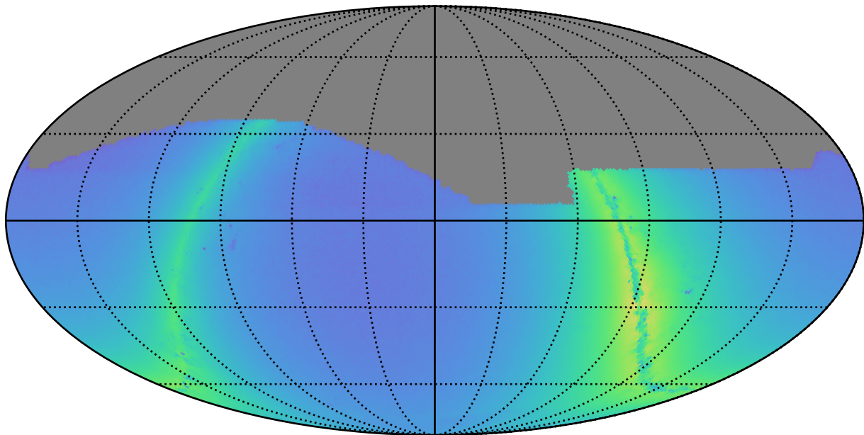
weather_cloudso18v3.4_10yrs z: Nstars_no_crowding
