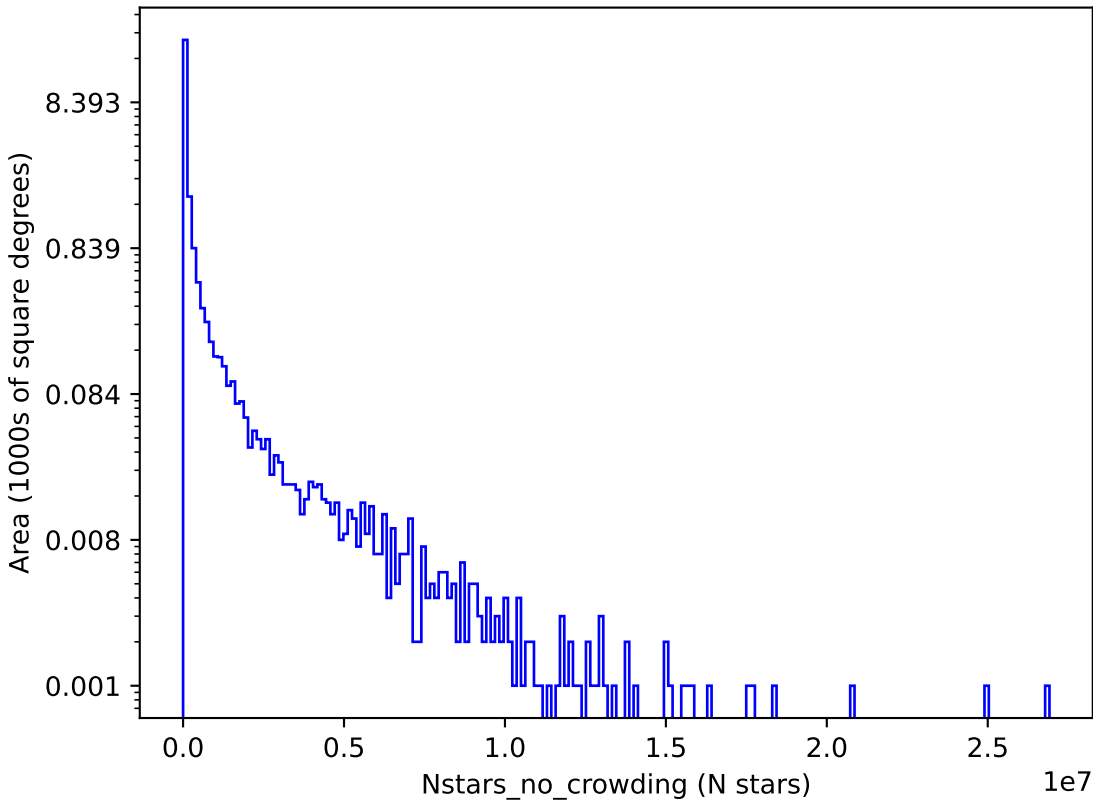
weather_cloudso18v3.4_10yrs z: Nstars_no_crowding
