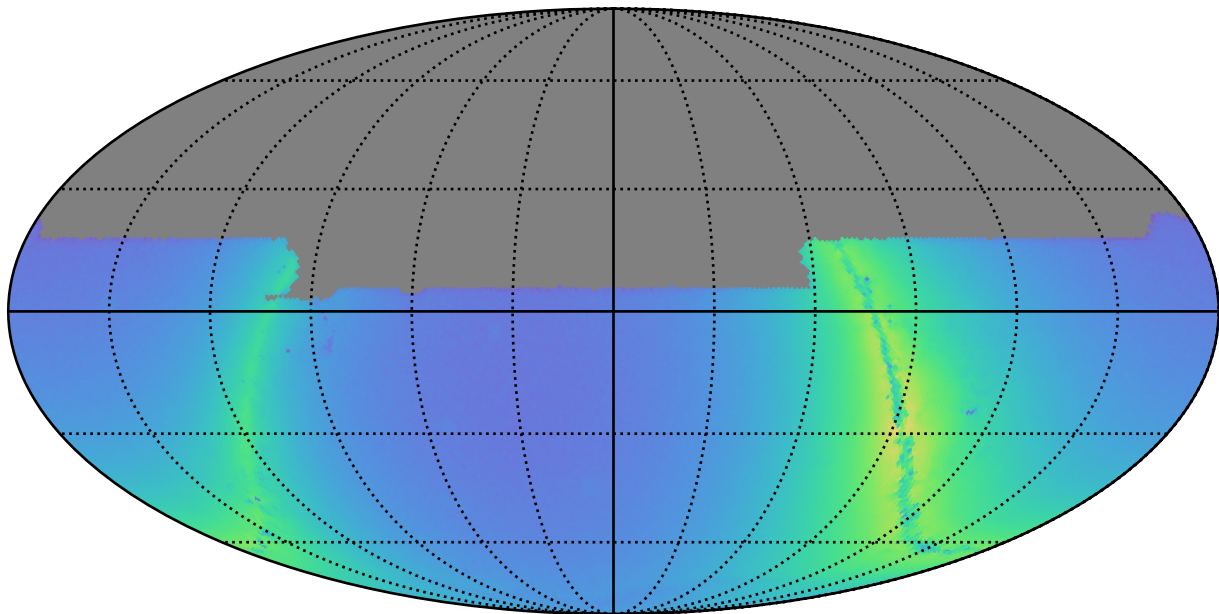
weather_cloudso18v3.4_10yrs y: Nstars_no_crowding
