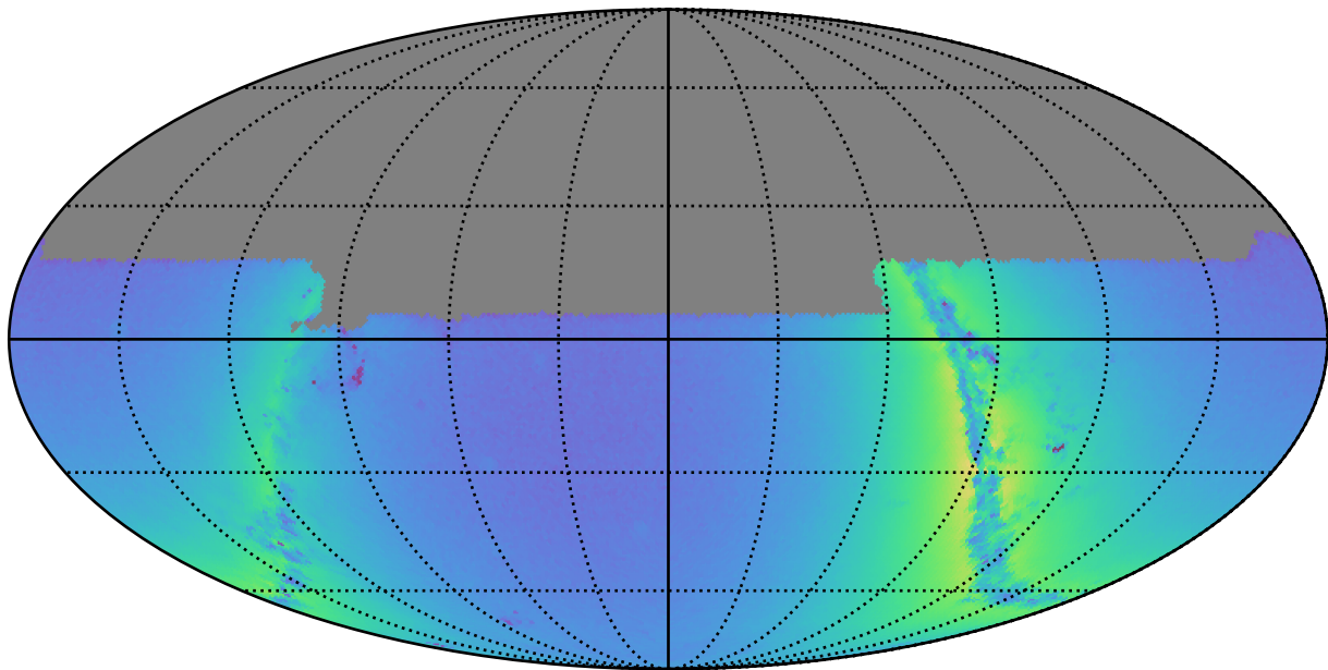
weather_cloudso18v3.4_10yrs u: Nstars_no_crowding
