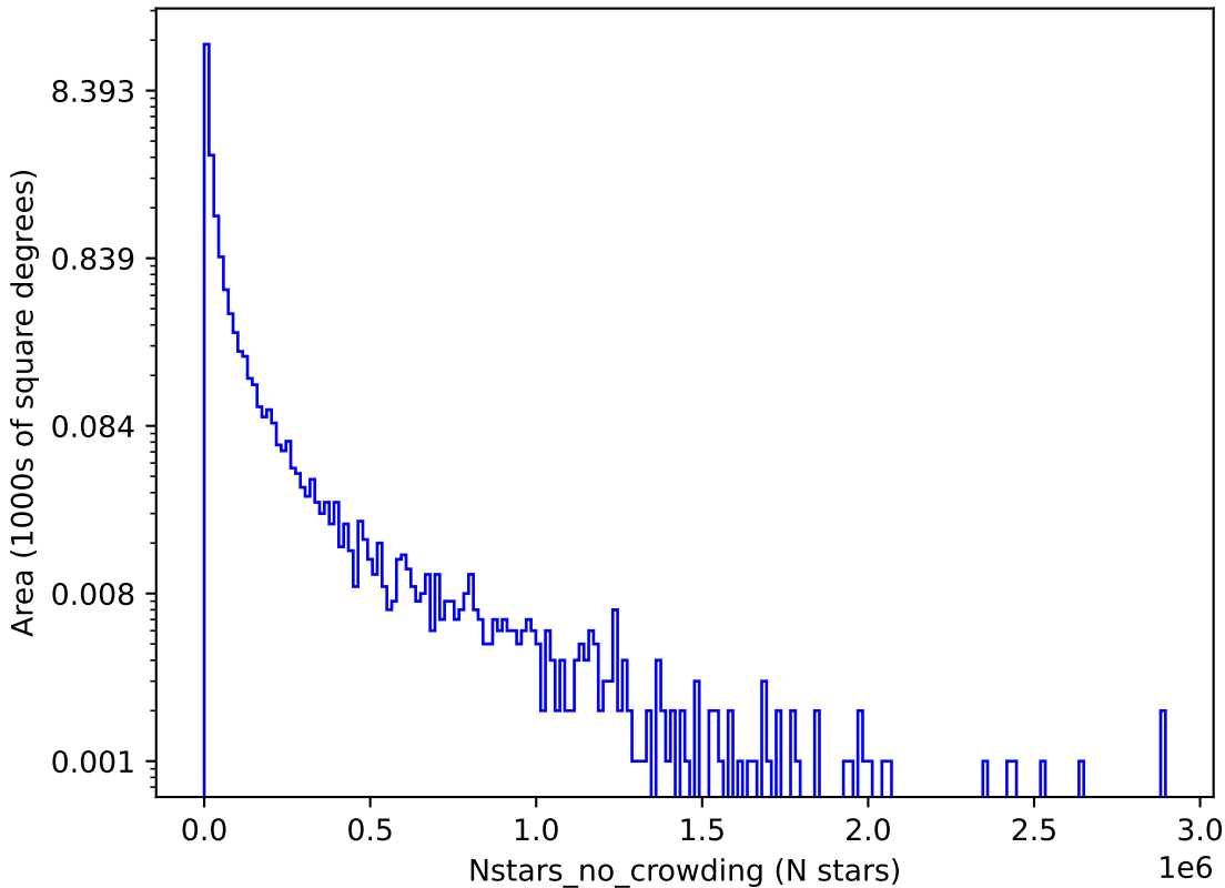
weather_cloudso18v3.4_10yrs u: Nstars_no_crowding
