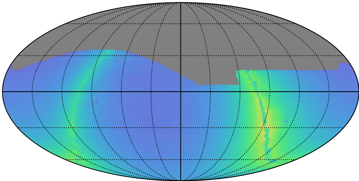
weather_cloudso18v3.4_10yrs r: Nstars_no_crowding
