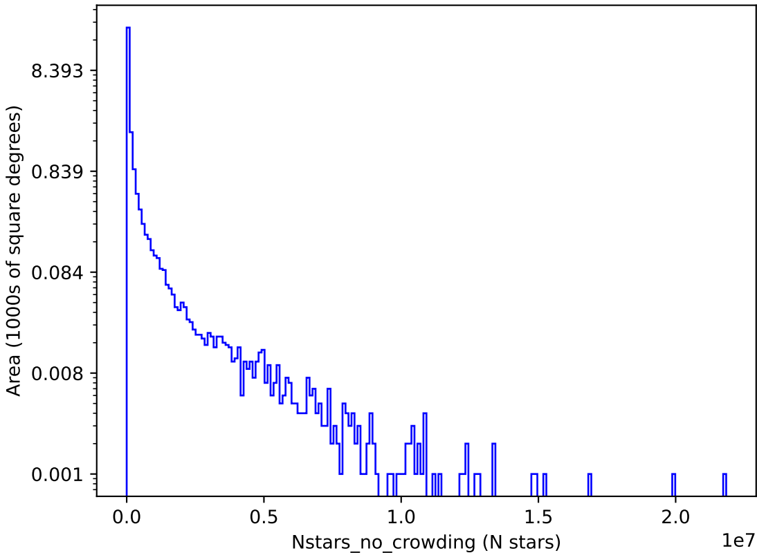
weather_cloudso18v3.4_10yrs r: Nstars_no_crowding
