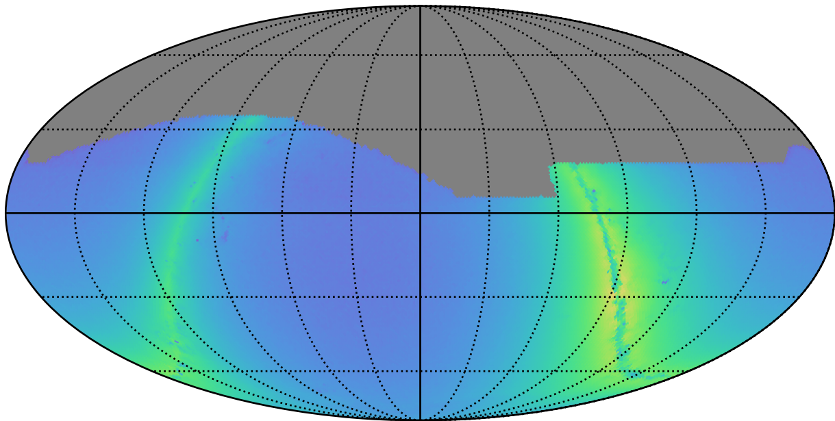
weather_cloudso18v3.4_10yrs i: Nstars_no_crowding
