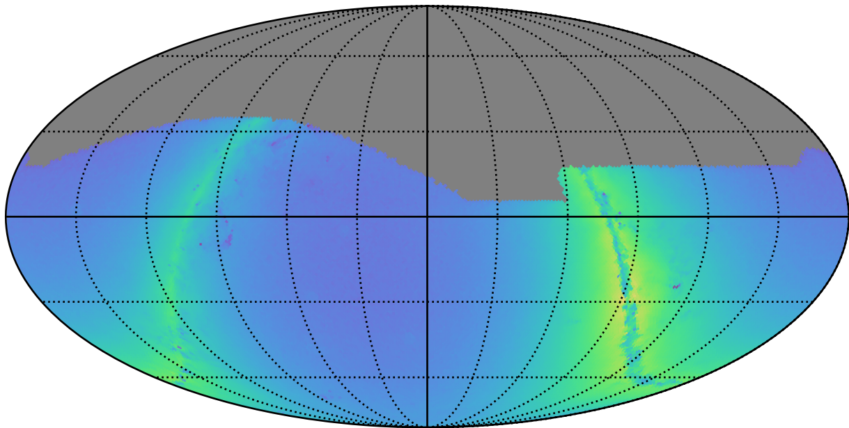
weather_cloudso18v3.4_10yrs g: Nstars_no_crowding
