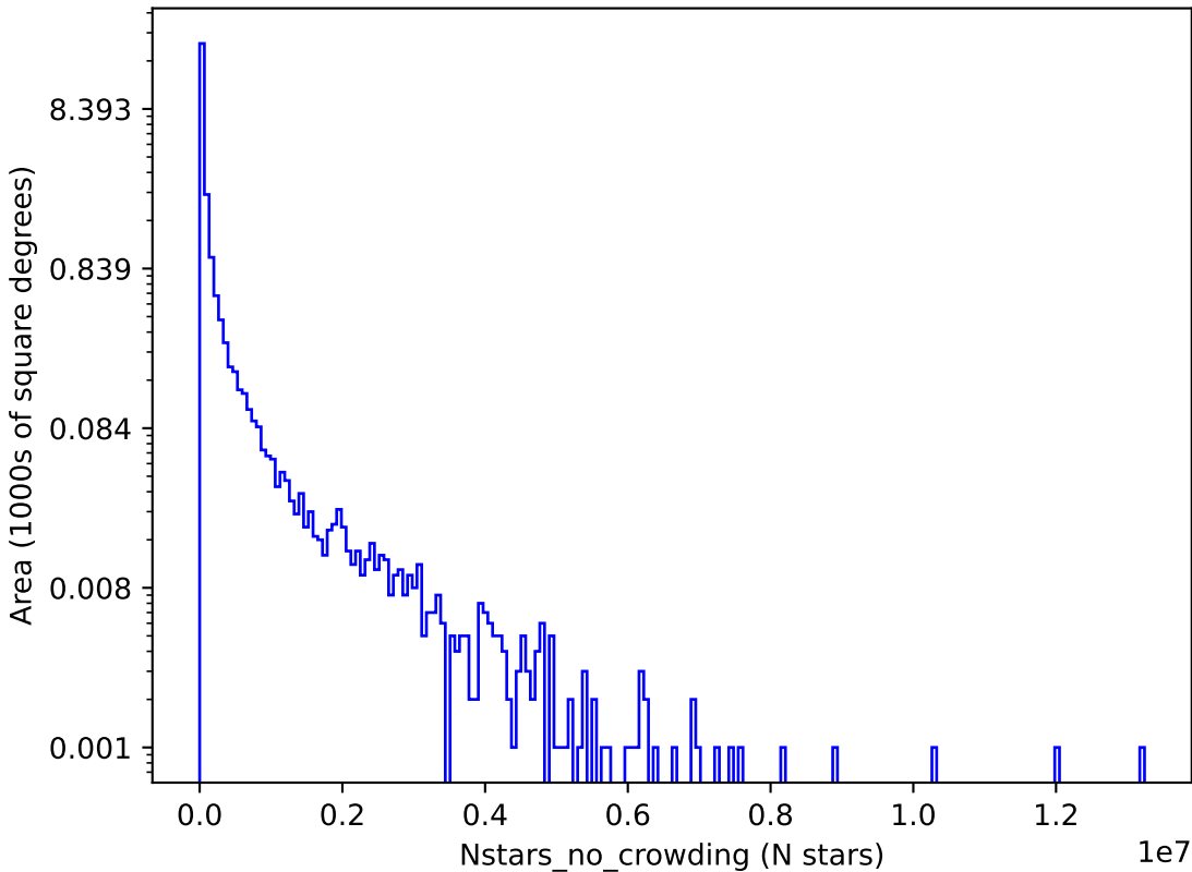
weather_cloudso18v3.4_10yrs g: Nstars_no_crowding
