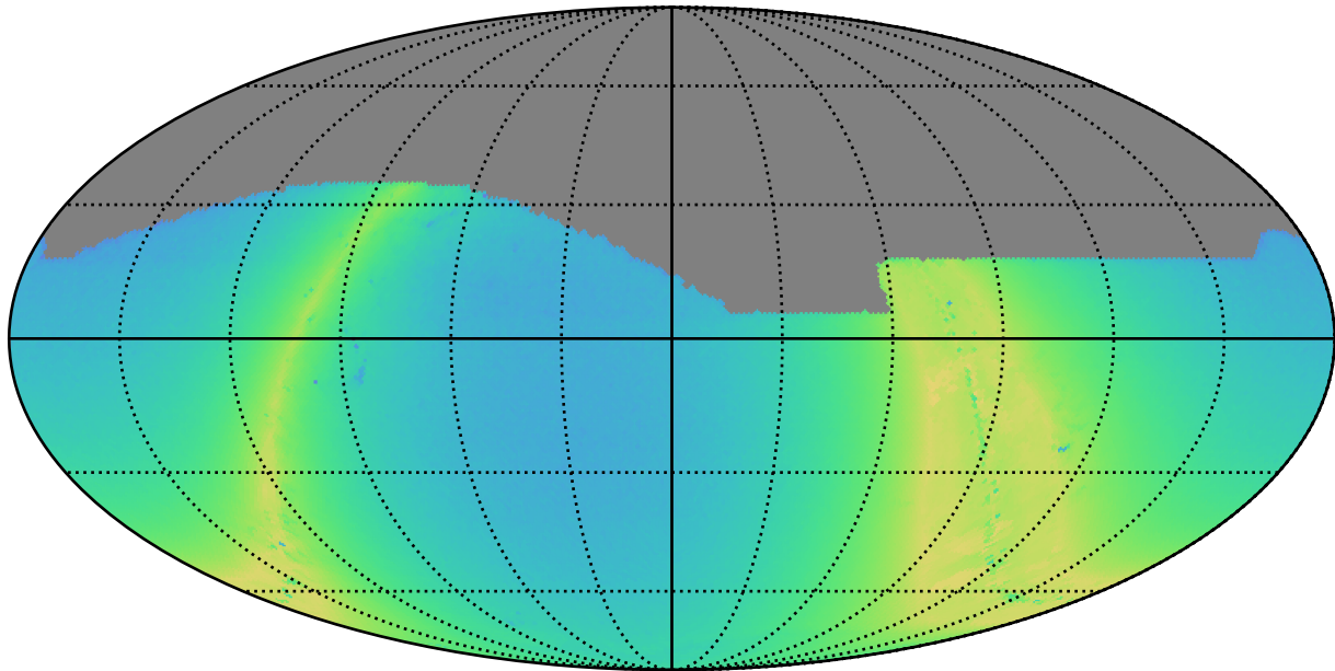
weather_cloudso18v3.4_10yrs i: N stars to Precision 0.20
