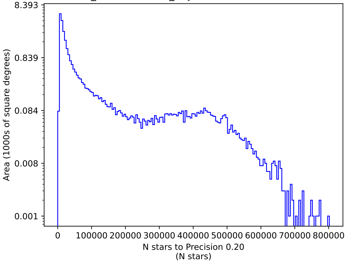
weather_cloudso18v3.4_10yrs i: N stars to Precision 0.20
