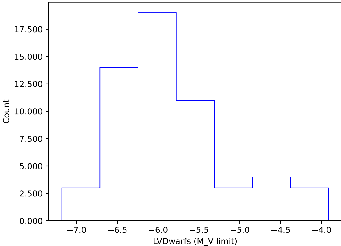
weather_cloudso18v3.4_10yrs gi: LVDwarfs
