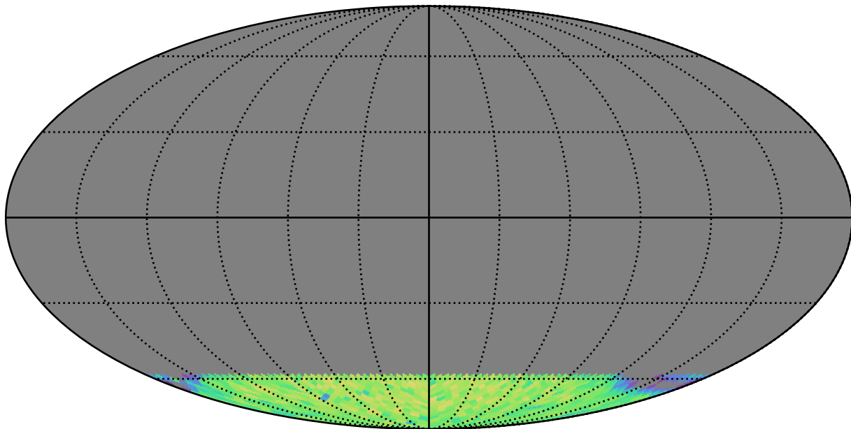
weather_cloudso18v3.4_10yrs gi SCP: LVDwarfs
