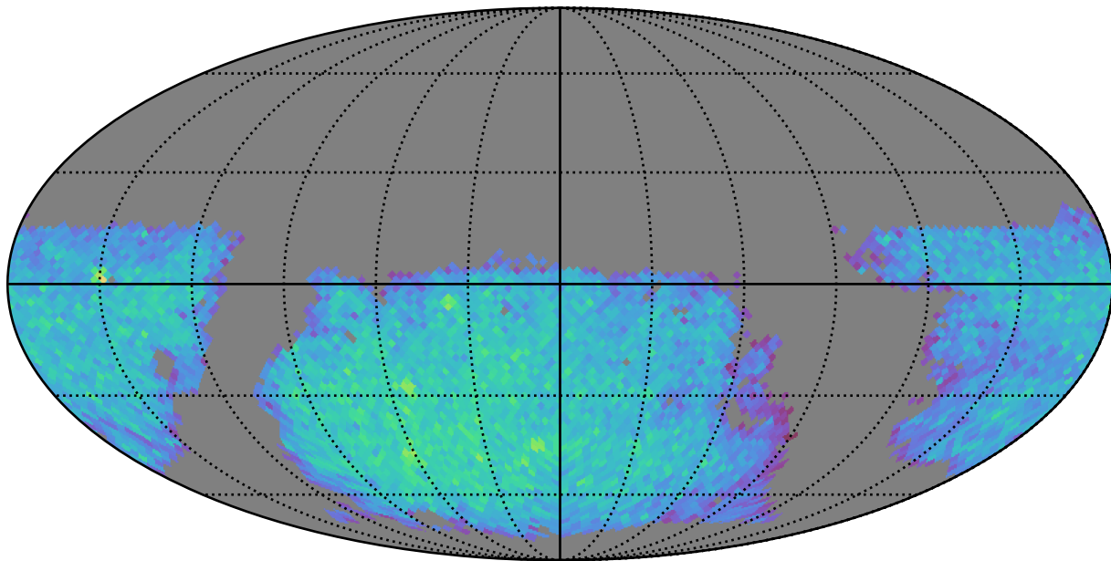
weather_cloudso18v3.4_10yrs gi: LVDwarfs
