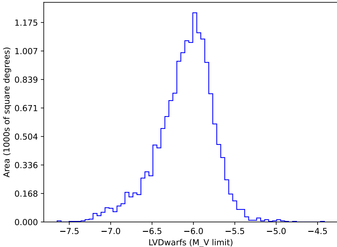
weather_cloudso18v3.4_10yrs gi: LVDwarfs
