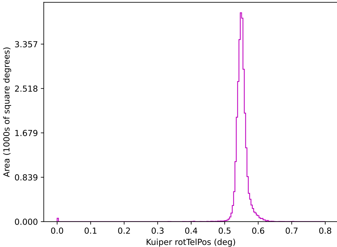
weather_cloudso18v3.4_10yrs z: Kuiper rotTelPos
