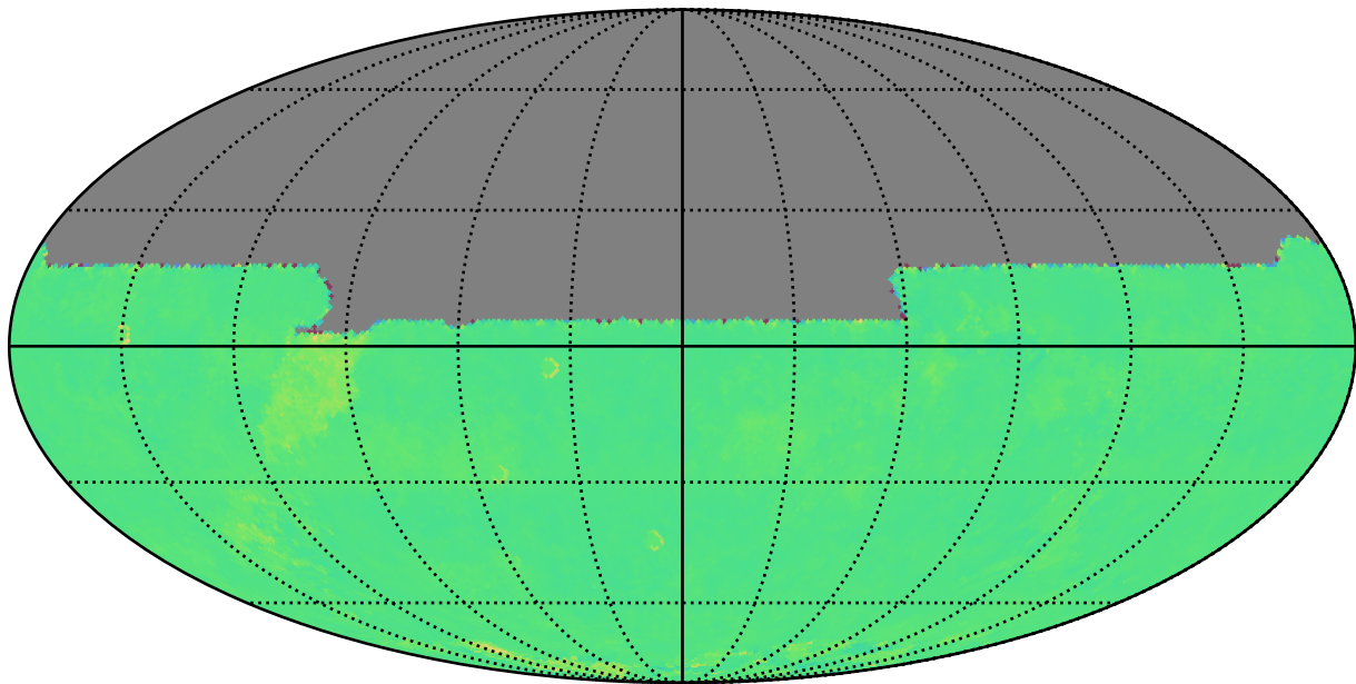
weather_cloudso18v3.4_10yrs y: Kuiper rotTelPos
