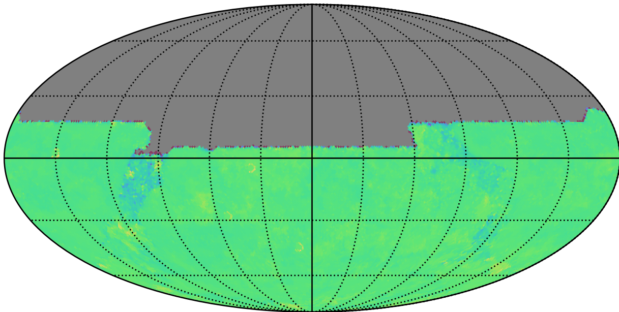
weather_cloudso18v3.4_10yrs u: Kuiper rotTelPos
