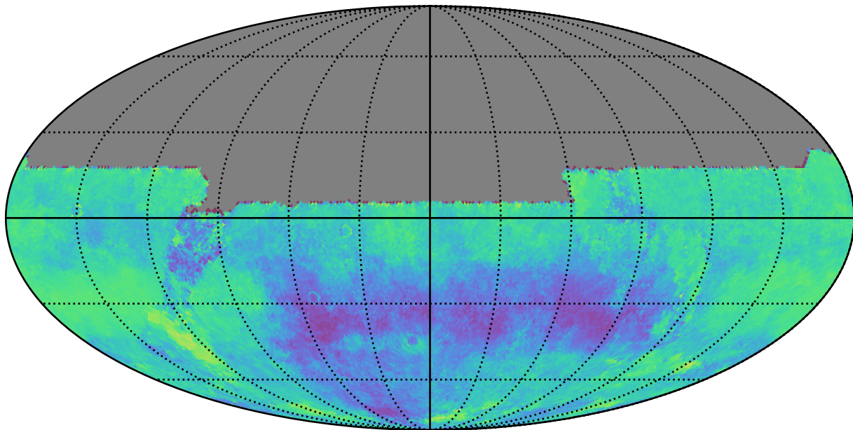
weather_cloudso18v3.4_10yrs u: Kuiper rotSkyPos
