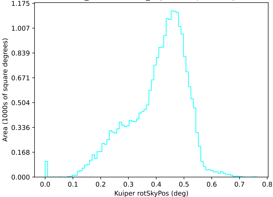
weather_cloudso18v3.4_10yrs u: Kuiper rotSkyPos
