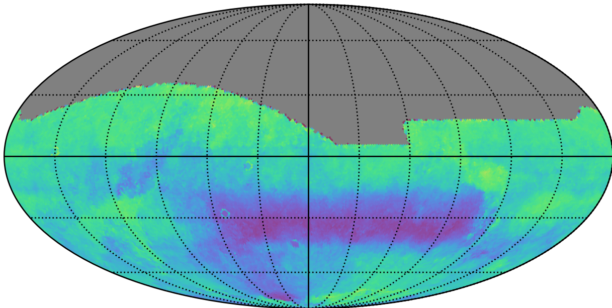
weather_cloudso18v3.4_10yrs r: Kuiper rotSkyPos
