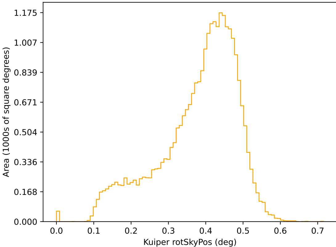
weather_cloudso18v3.4_10yrs r: Kuiper rotSkyPos
