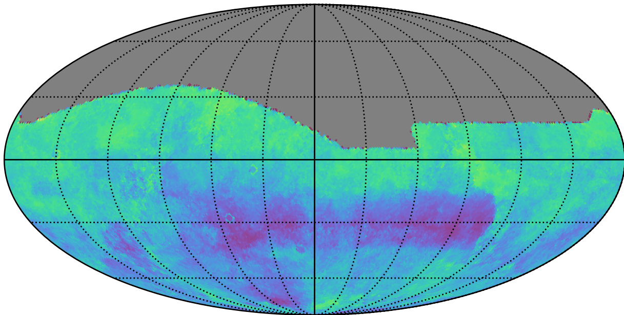
weather_cloudso18v3.4_10yrs g: Kuiper rotSkyPos
