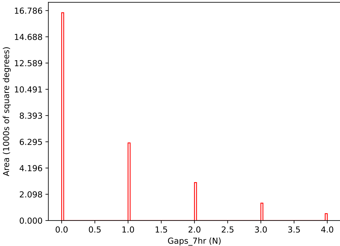
weather_cloudso18v3.4_10yrs i band: Gaps_7hr
