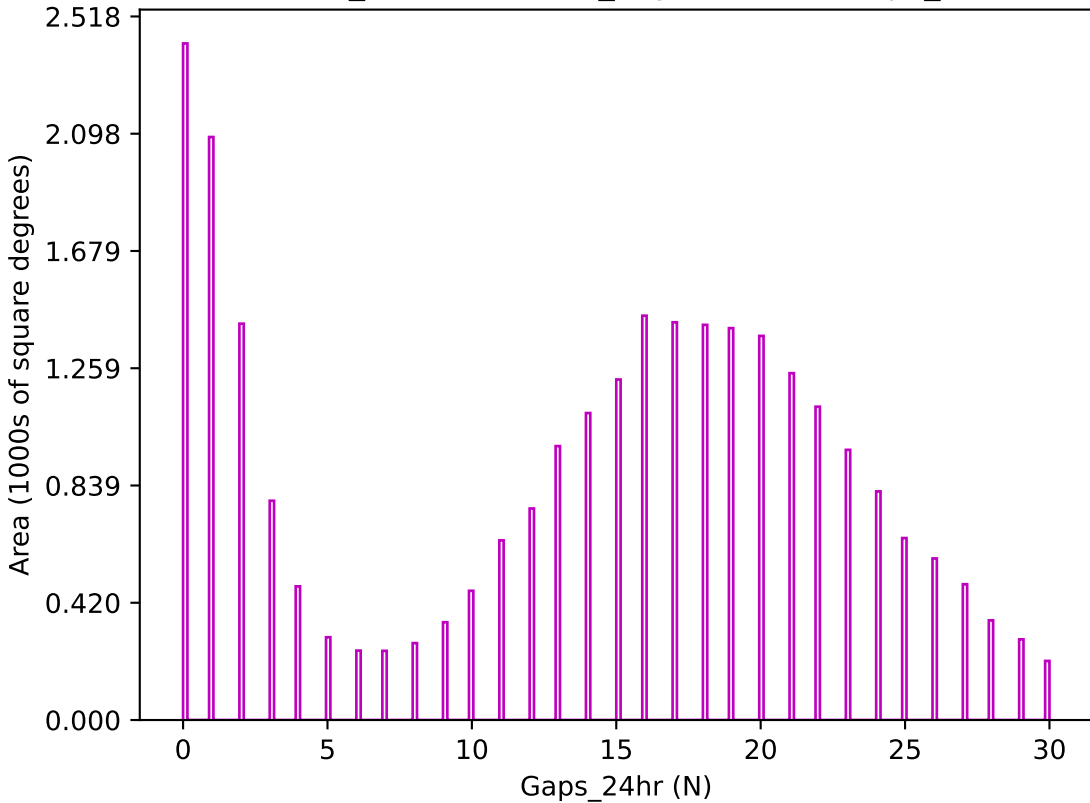
weather_cloudso18v3.4_10yrs z band: Gaps_24hr
