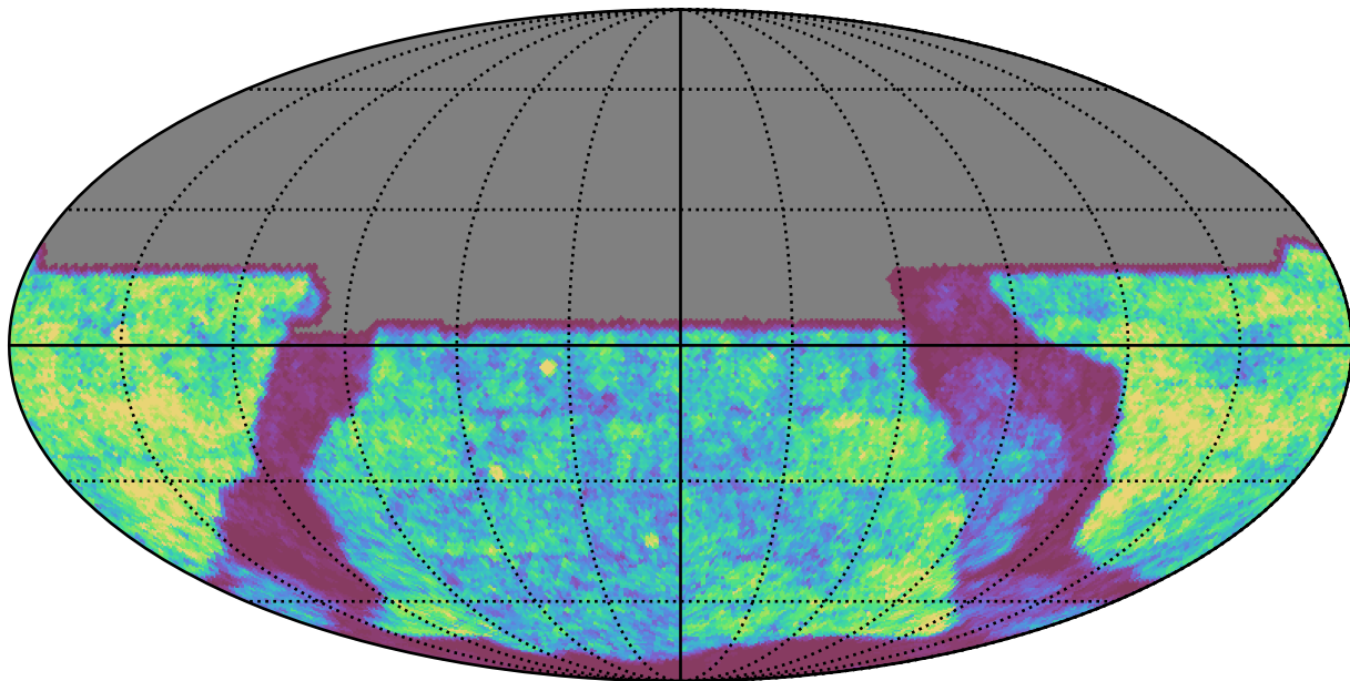
weather_cloudso18v3.4_10yrs y band: Gaps_24hr
