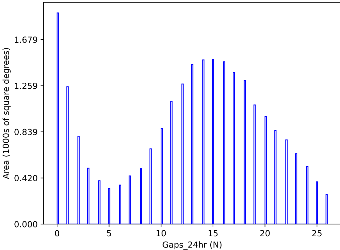
weather_cloudso18v3.4_10yrs y band: Gaps_24hr
