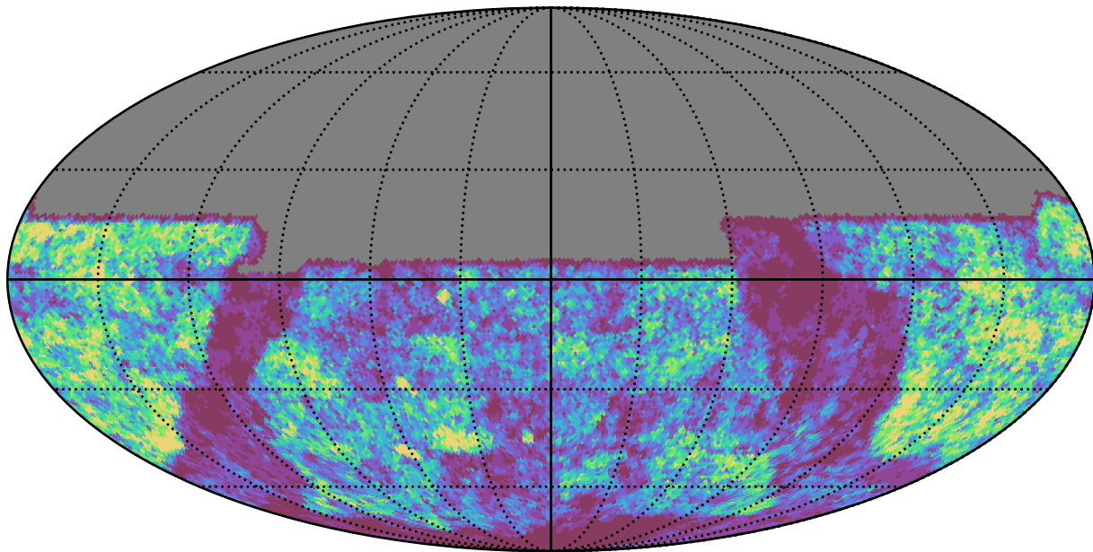
weather_cloudso18v3.4_10yrs u band: Gaps_24hr
