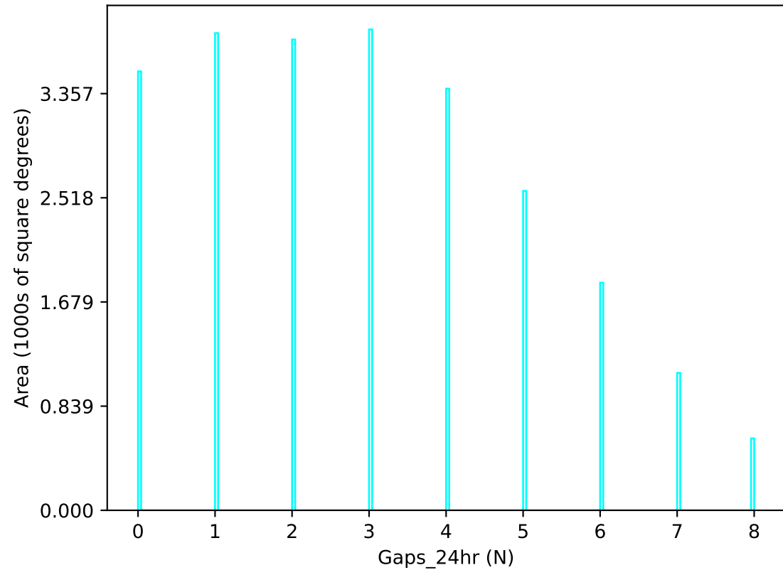
weather_cloudso18v3.4_10yrs u band: Gaps_24hr
