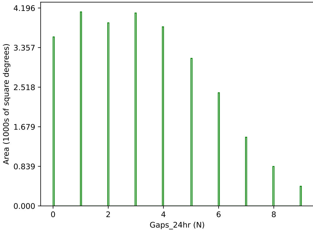
weather_cloudso18v3.4_10yrs g band: Gaps_24hr
