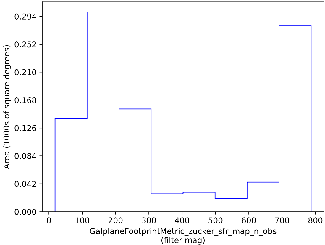
weather_cloudso18v3.4_10yrs : GalplaneFootprintMetric_zucker_sfr_map_n_obs
