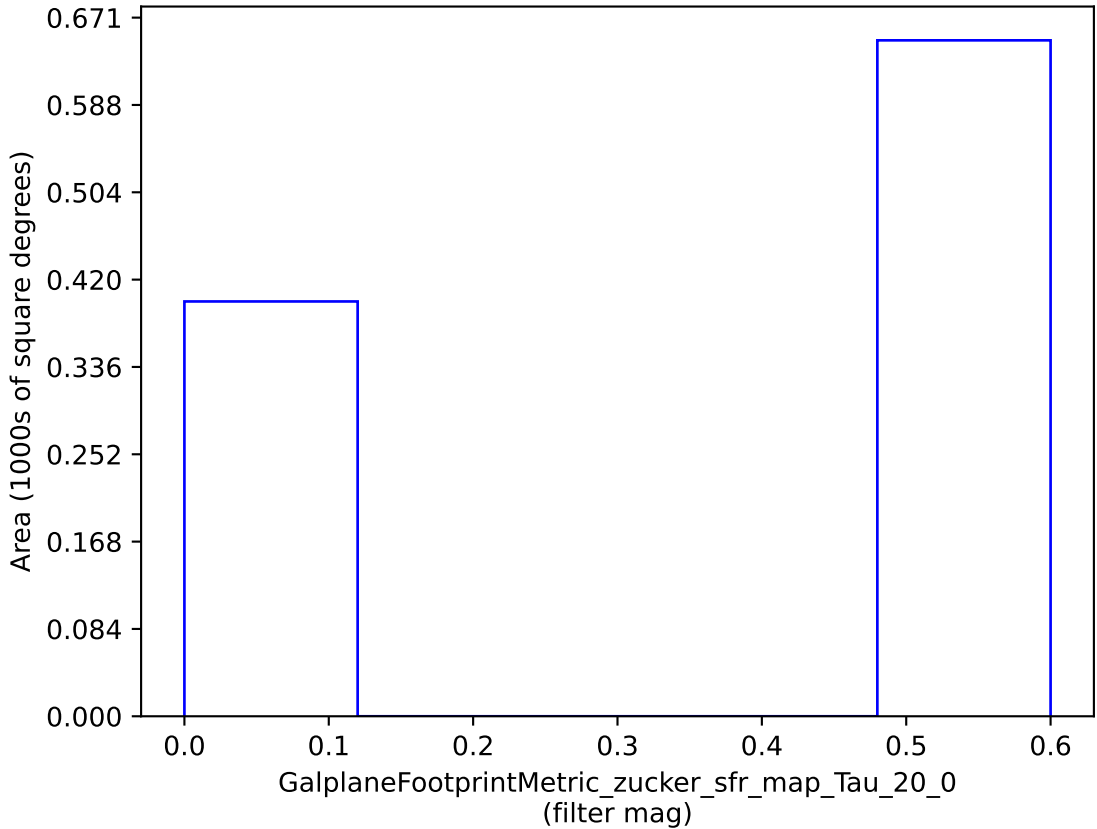
weather_cloudso18v3.4_10yrs : GalplaneFootprintMetric_zucker_sfr_map_Tau_20_0
