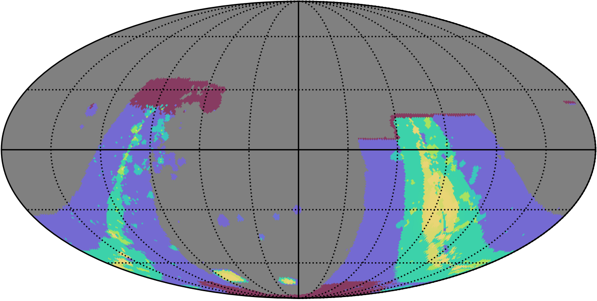
weather_cloudso18v3.4_10yrs : GalplaneFootprintMetric_combined_map_Tau_46_5
