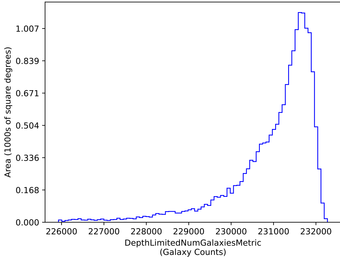
weather_cloudso18v3.4_10yrs i band galaxies non-DD: DepthLimitedNumGalaxiesMetric
