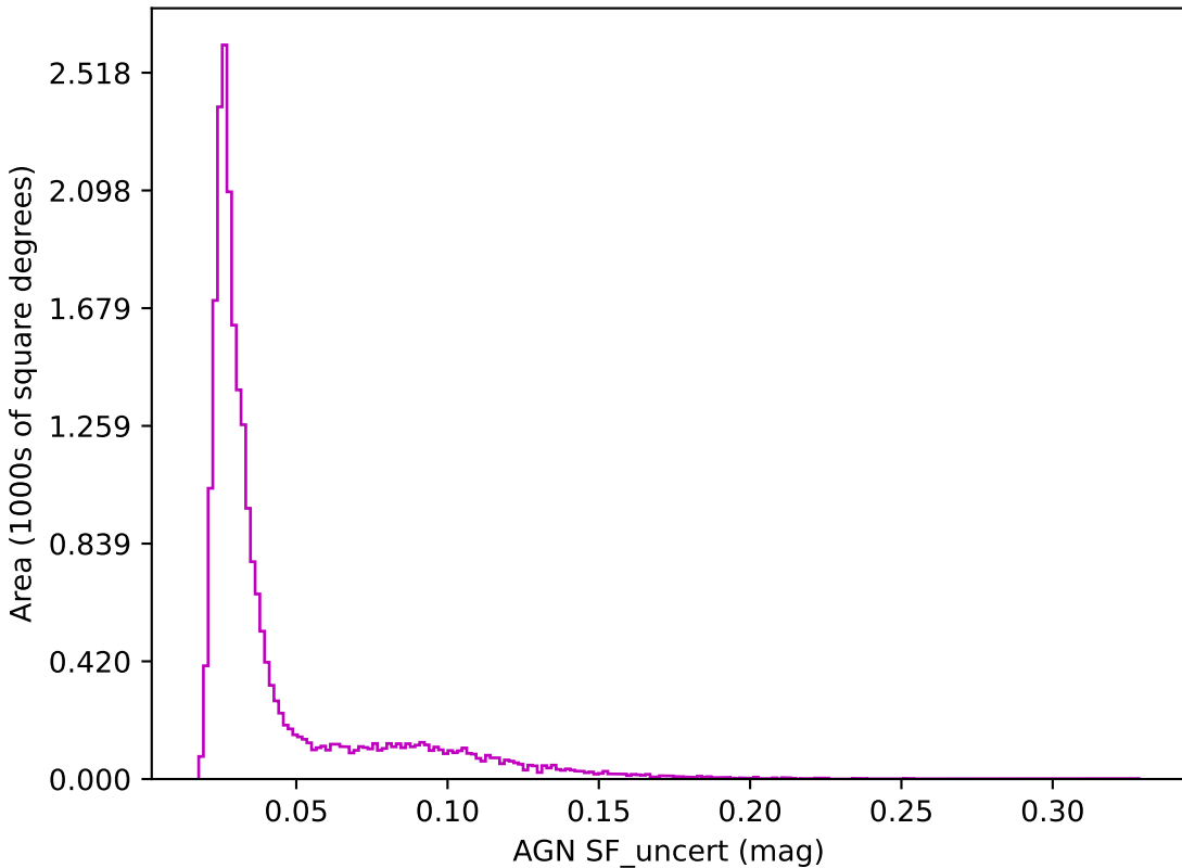
weather_cloudso18v3.4_10yrs z band: AGN SF_uncert
