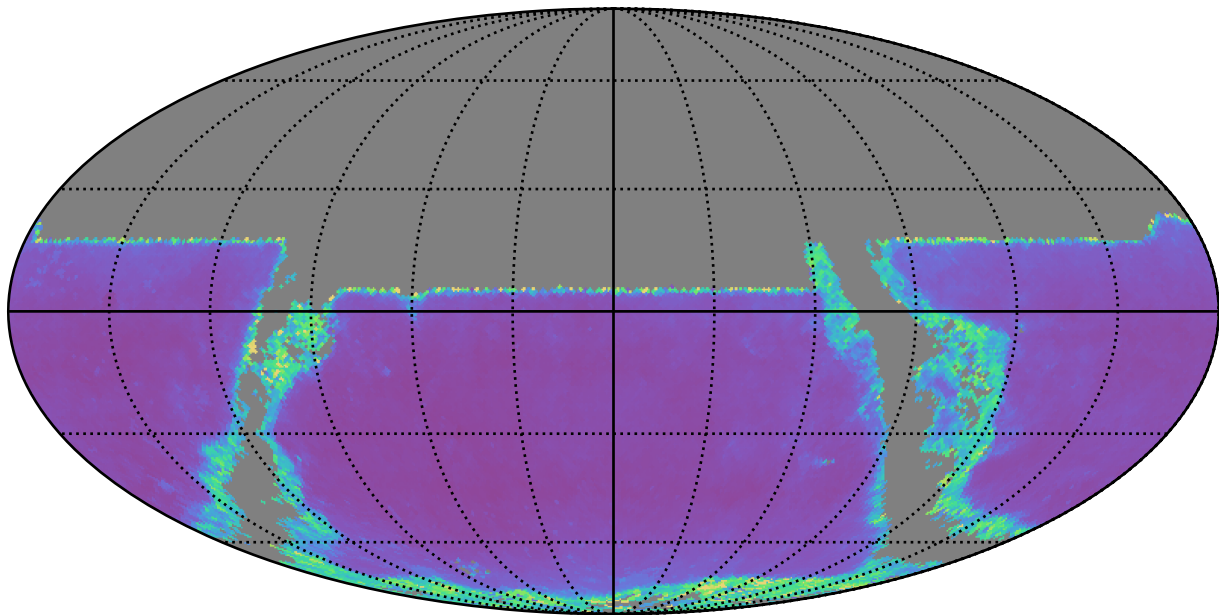
weather_cloudso18v3.4_10yrs y band: AGN SF_uncert
