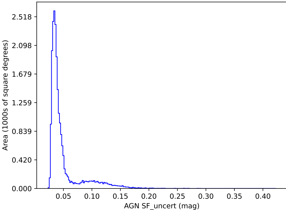
weather_cloudso18v3.4_10yrs y band: AGN SF_uncert
