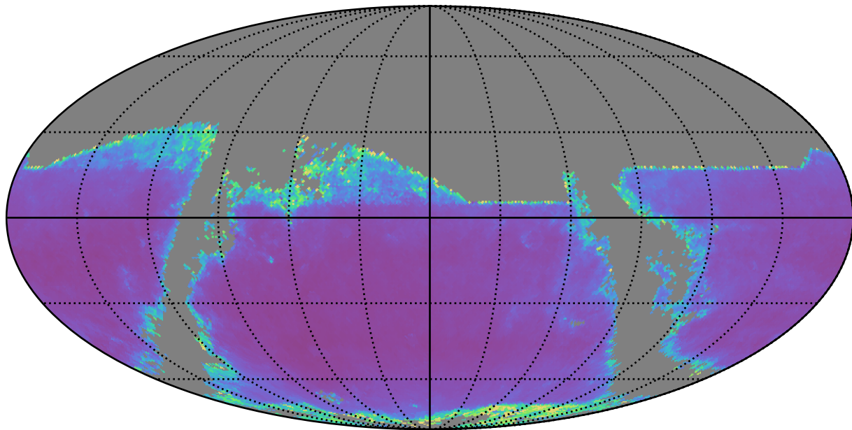
weather_cloudso18v3.4_10yrs r band: AGN SF_uncert
