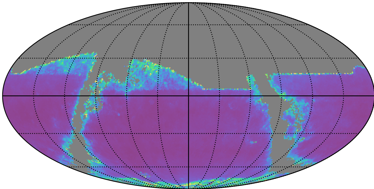
weather_cloudso18v3.4_10yrs i band: AGN SF_uncert
