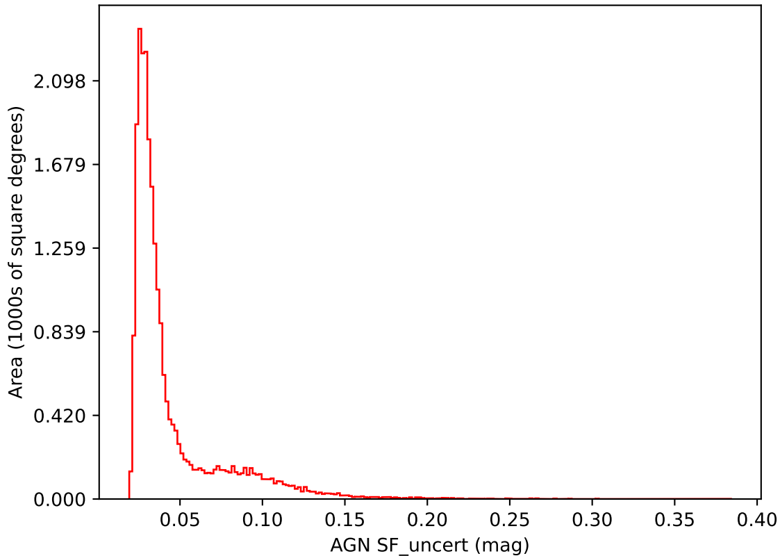
weather_cloudso18v3.4_10yrs i band: AGN SF_uncert
