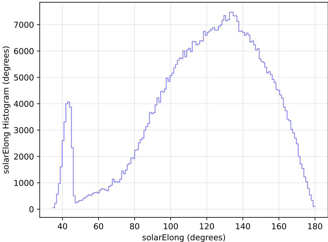
weather_cloudso18v3.4_10yrs WFD i band: solarElong Histogram
