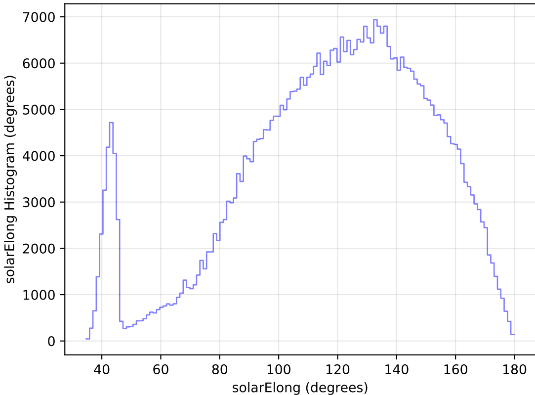
weather_cloudso18v3.4_10yrs All sky z band: solarElong Histogram
