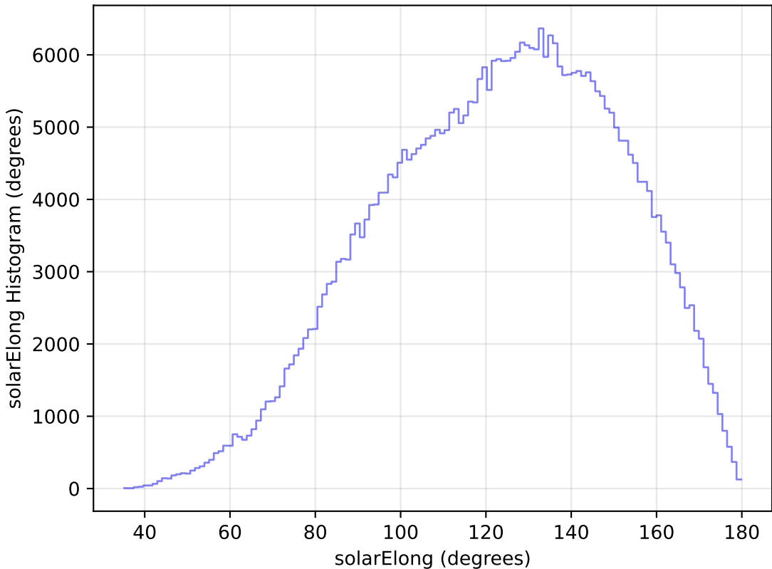
weather_cloudso18v3.4_10yrs All sky y band: solarElong Histogram
