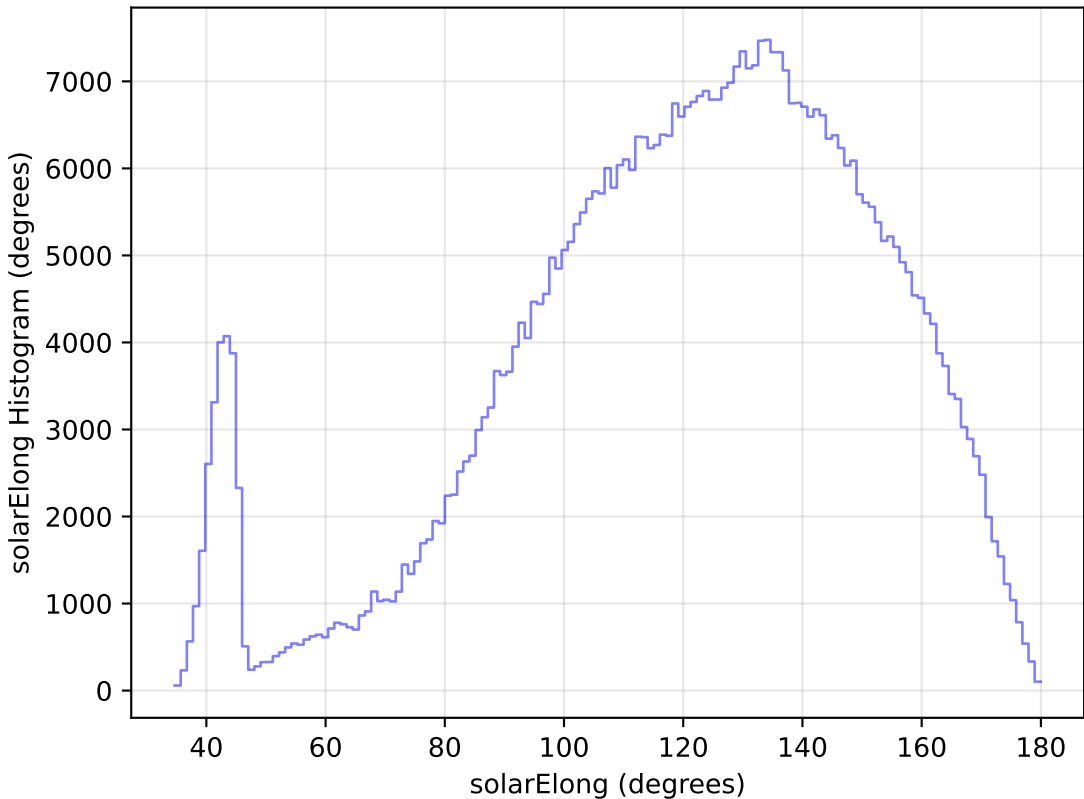
weather_cloudso18v3.4_10yrs All sky i band: solarElong Histogram
