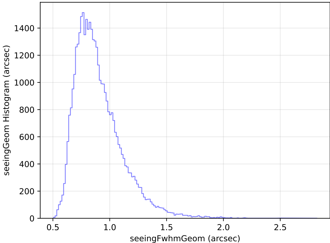
weather_cloudso18v3.4_10yrs Yr 1 y band: seeingGeom Histogram
